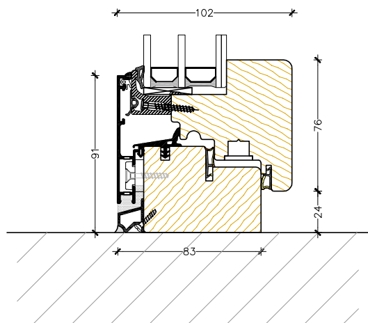
Nodo basso finestra
