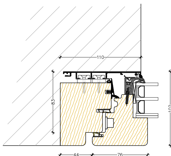
Nodo laterale e alto complanare interno ed esterno
