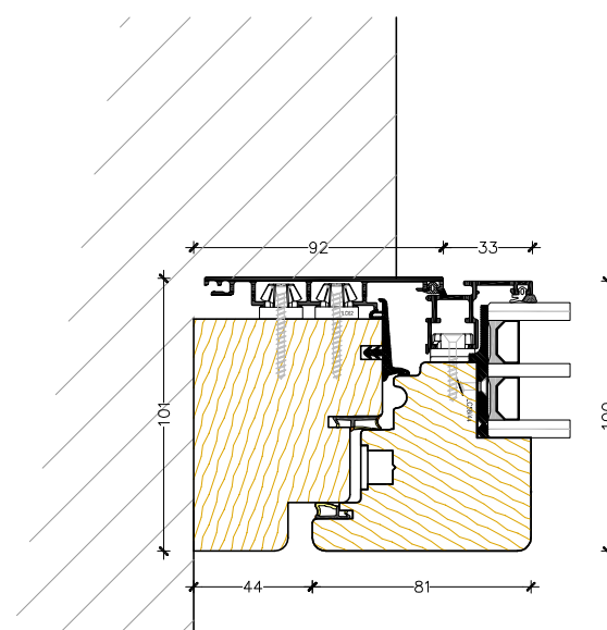
Nodo laterale e alto complanare interno ed esterno
