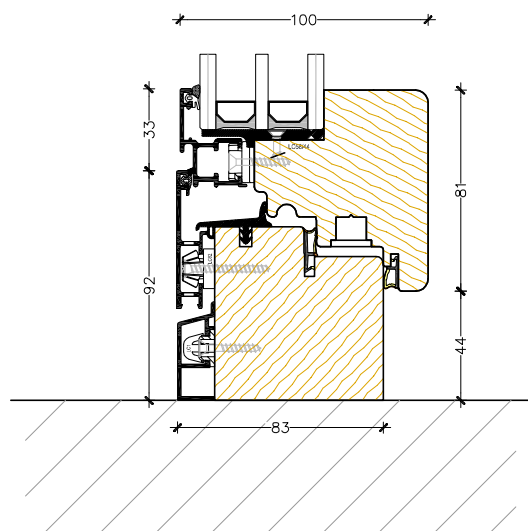
Nodo basso finestra
